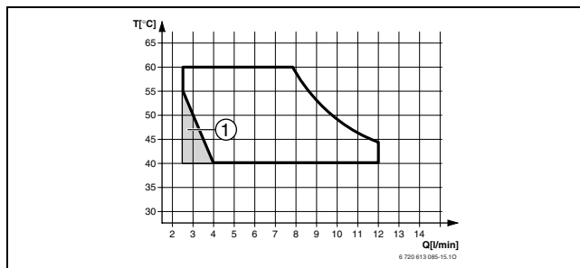
Sl. 11 Dijagram za ulaznu temperaturu hladne vode od +15 °C (ZWC 24-3 MFA/MFK)
